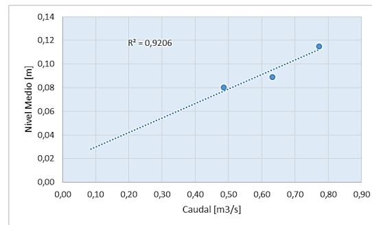
Figura 15. Relación Nivel Medio vs Caudal 2016
