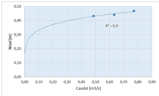
Figura 16. Curva de Calibración Estación El Rasgón 2016
