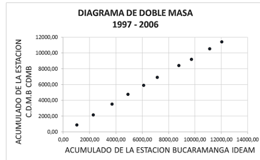
Figura 6. Grafica de Doble Masa Estación CDMB y Estación Bucaramanga IDEAM
