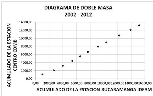
Figura 4. Grafica de Doble Masa Estación Centro y Estación Bucaramanga IDEAM
