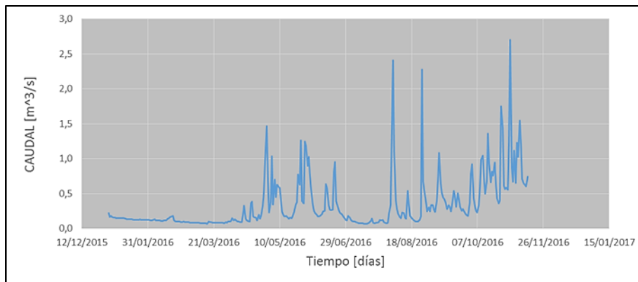
Figura 17. Caudal Medio Diario 2016
