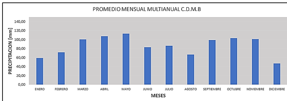
Figura 8. Promedio mensual Multianual Estación CDMB 1979 – 2006
