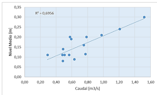
Figura 14. Relación Nivel Medio vs Caudal 2012 – 2016
