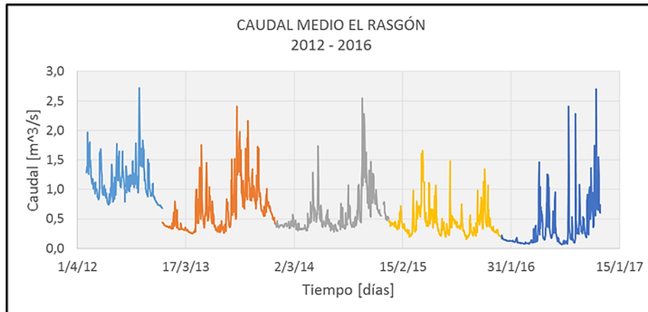
Figura 18. Caudal Medio Diario 2012 - 2016
