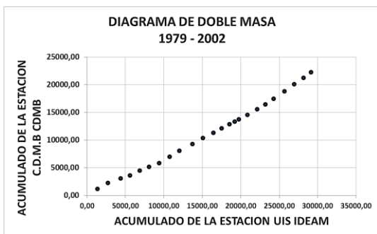
Figura 5. Grafica de Doble Masa Estación CDMB y Estación UIS IDEAM
